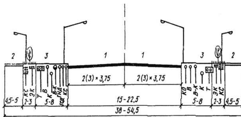
Рис. 5. Типовые поперечные профили магистралей районного значения
